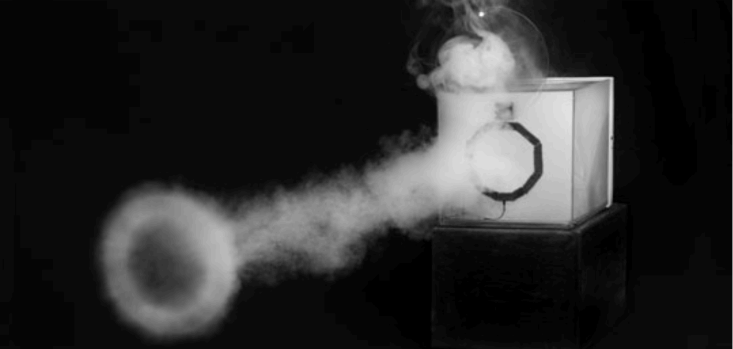
Máquinas de fumaça, 2010-2011; duas caixas acrílicas de 65x50cm, membrana plástica, reservatório de líquido, máquinas de fumaça, disparador, solenoide e Programmable Interface Controller — PIC, coleção da artista
